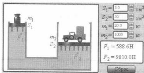
Рис. 5.15. Компьютерная визуальная интерактивная модель гидравлической машины
