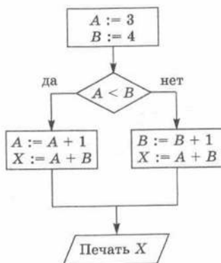
Рис. 5.10. Информационная модель — блок-схема алгоритма
