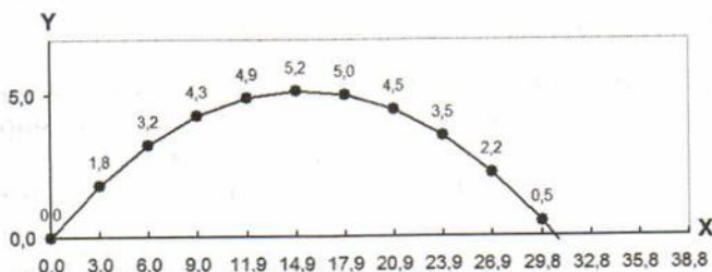
Рис. 5.1.3. Траектория движения мячика
