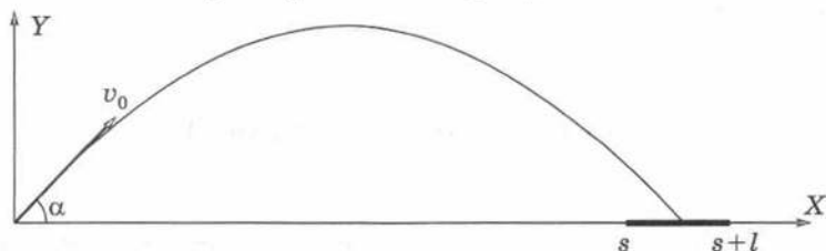
Рис. 5.16. Бросание мячика в площадку
