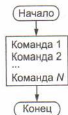
Рис. 4.2. Линейный алгоритм
