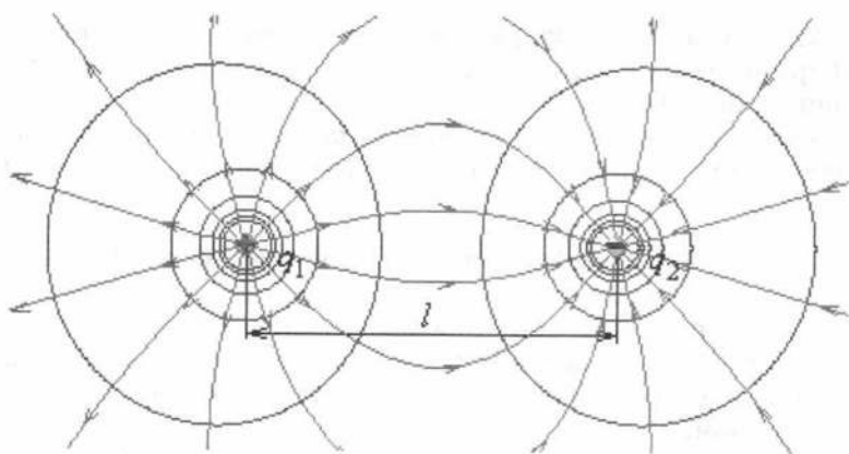
Рис. 5.13. Описательная модель взаимодействия электрических зарядов
