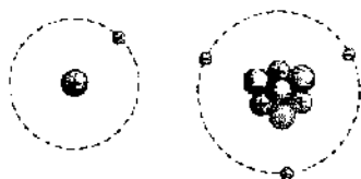
Рис. 5.4. Атом водорода и атом лития
