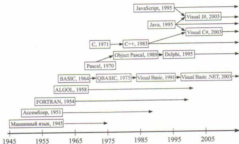
Рис. 4.1. История развития языков программирования
