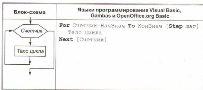
Рис. 4.5. Алгоритмическая структура «цикл со счетчиком»
