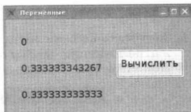
Рис. 4.2.2. Проект «Переменные» на языке Gambas
