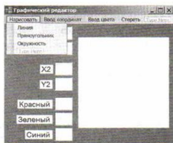
Рис. 4.10.1. Создание меню графического редактора
