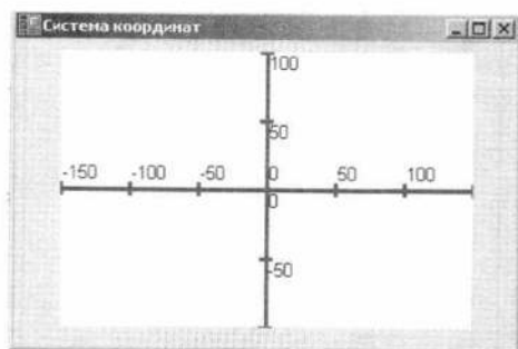
Рис. 4.11. Математическая система координат графического поля
