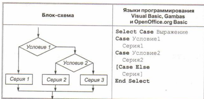
Рис. 4.4. Алгоритмическая структура «выбор»
