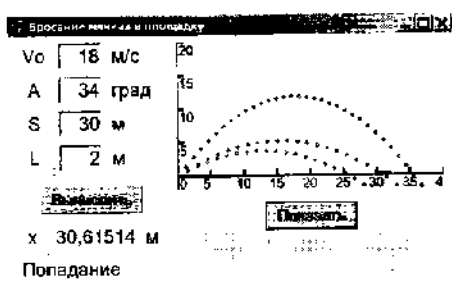
Рис. 5.1.1. Проект «Бросание мячика в площадку» на языке Visual Basic
